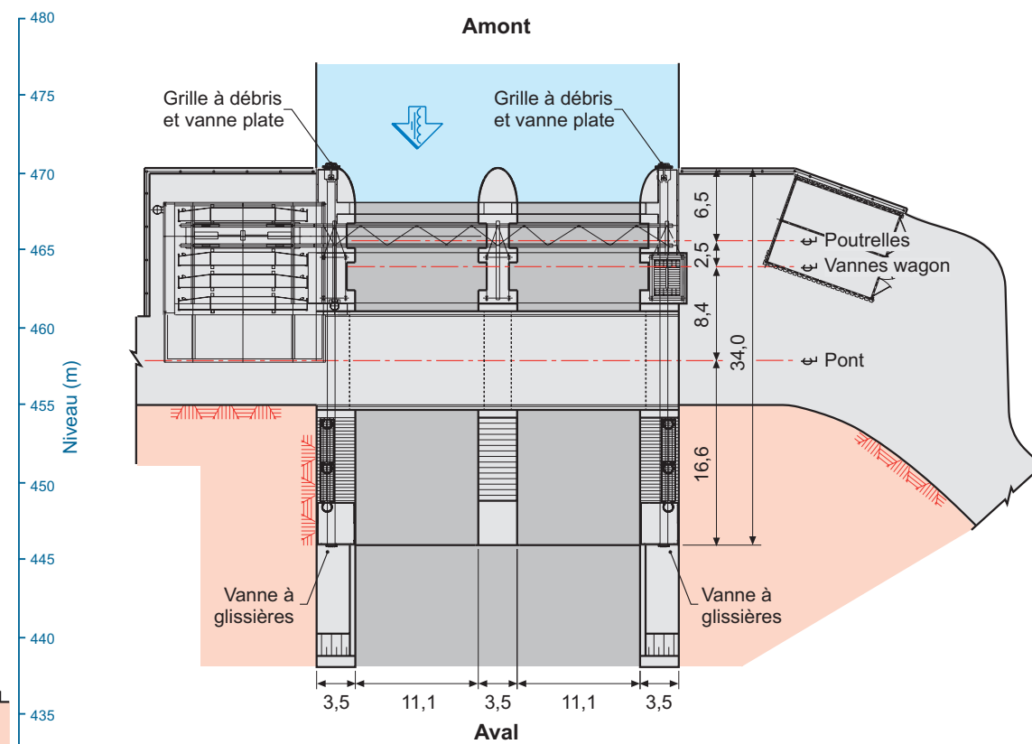
Évacuateur de crues – Vue en plan
