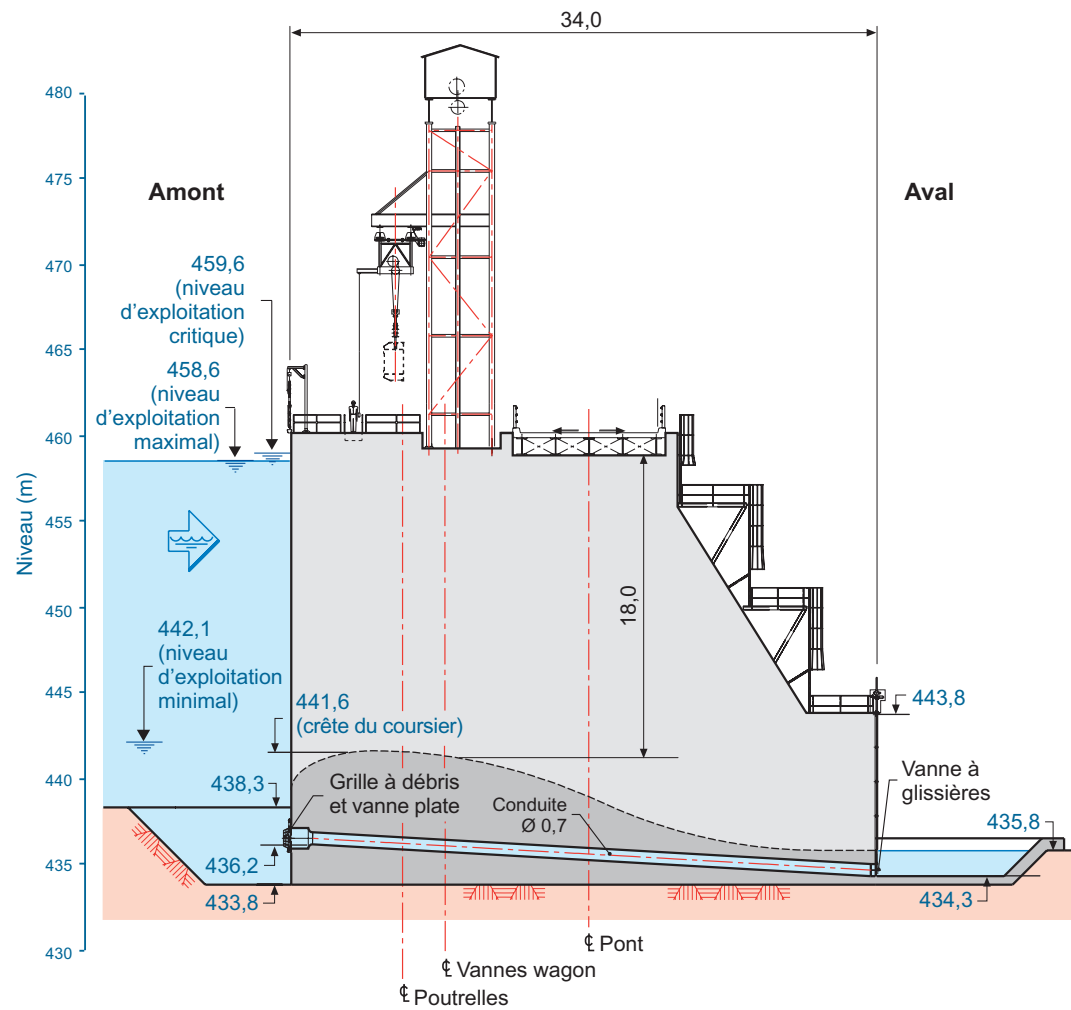
Évacuateur de crues – Détail
