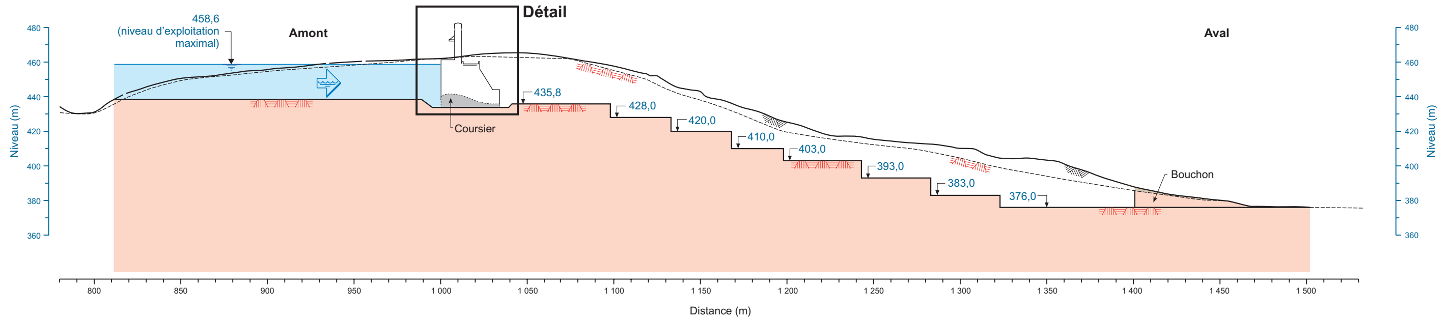
Évacuateur de crues – Profil longitudinal A
